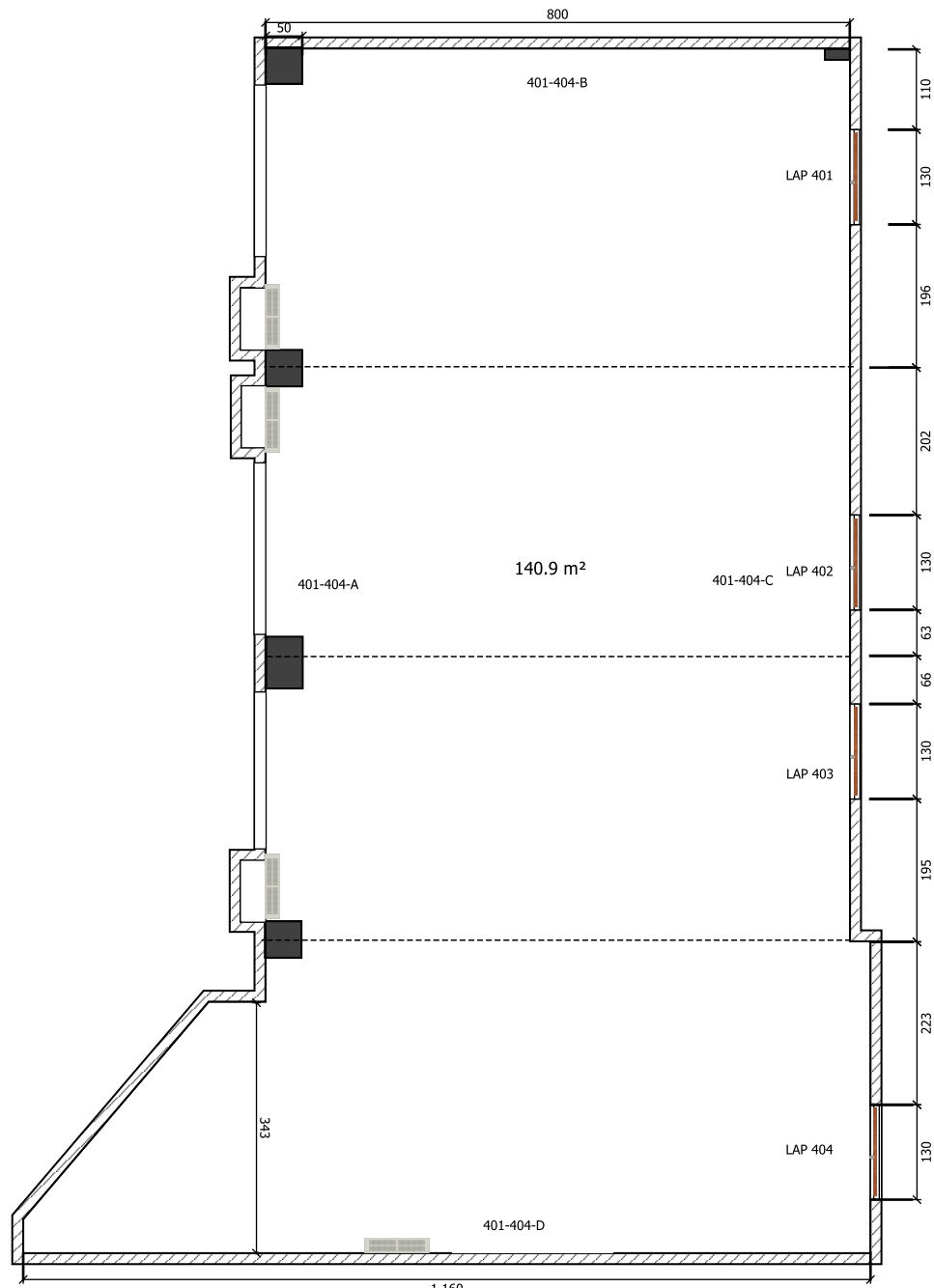
RUANG LAP 401--404 SKALA 1:100
